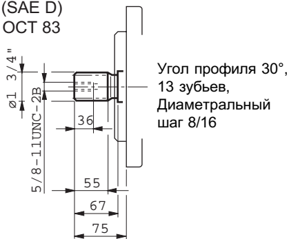
Вид W
